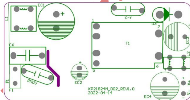
Top Layer
