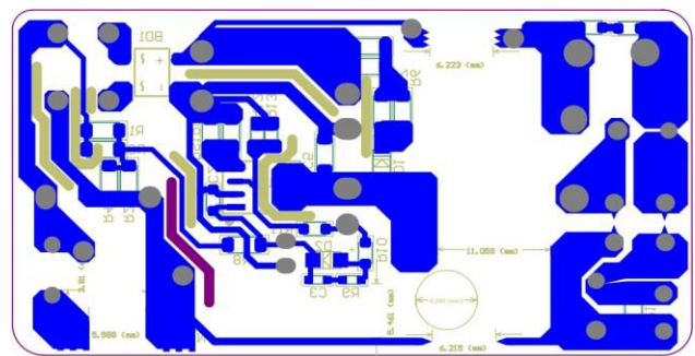
Bottom Layer
